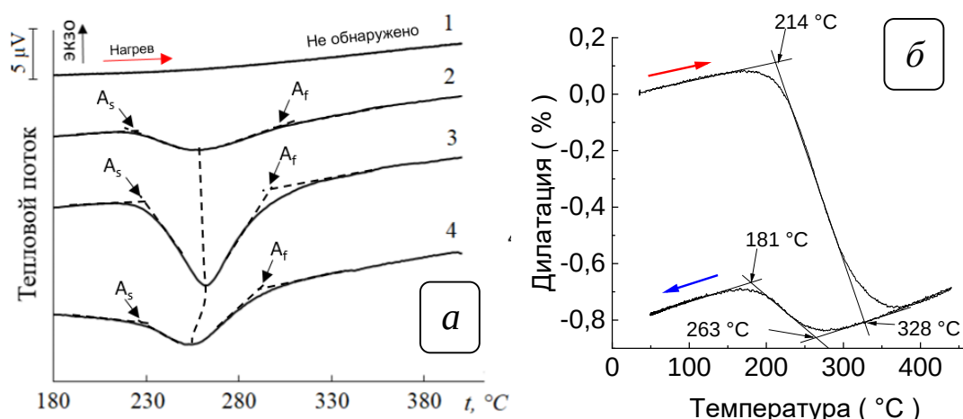
Рисунок 3.12 – ДСК-кривые, полученные при нагревании: 1 – спекание 1250 °C, 2 часа; 2 – спекание 1300 °C, 3 часа; 3 – спекание 1300 °C, 3 часа + отжиг 1000 °C, 4 часа; 4 – спекание 1300 °C, 3 часа + отжиг 1000 °C, 16 часов (а); дилатометрия образца после спекания 1250 °C, 2 часа (б)
