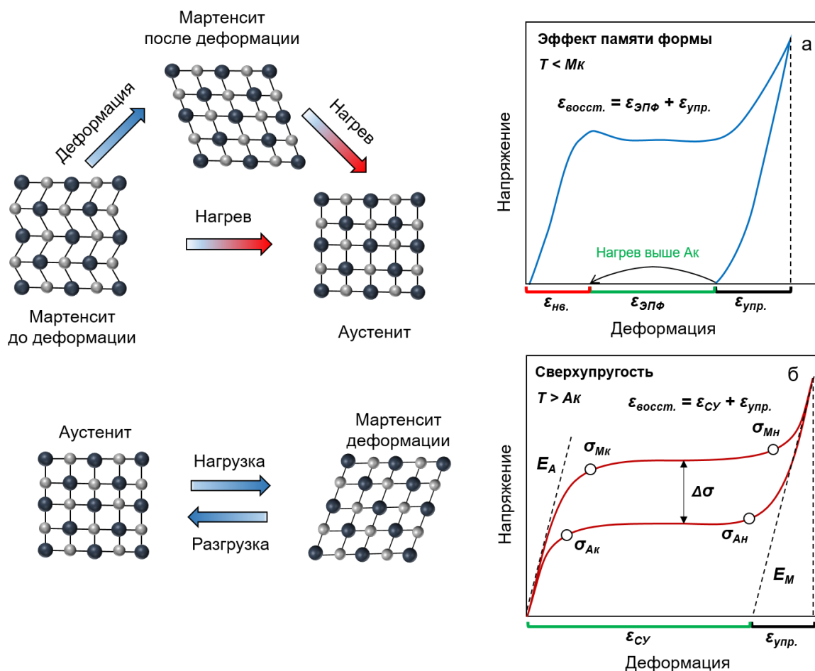
Рисунок 1.2 – Схематическое изображение эффекта памяти формы (ЭПФ) и суперупругости (СУ)
