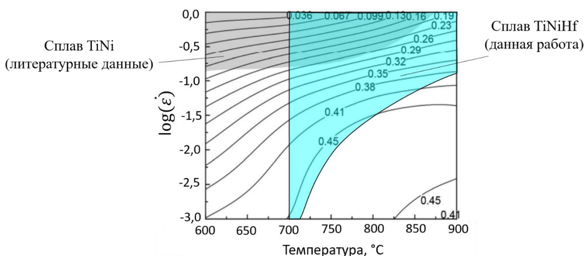
Рисунок 4.10 – Карта деформации сплава Ti-(55,85-56,05)Ni % мас. Серая и голубая области – области неустойчивости пластического течения ( \xi -критерий < 0 ) бинарного сплава TiNi [103] и сплава TiNiHf (настоящая работа) соответственно
