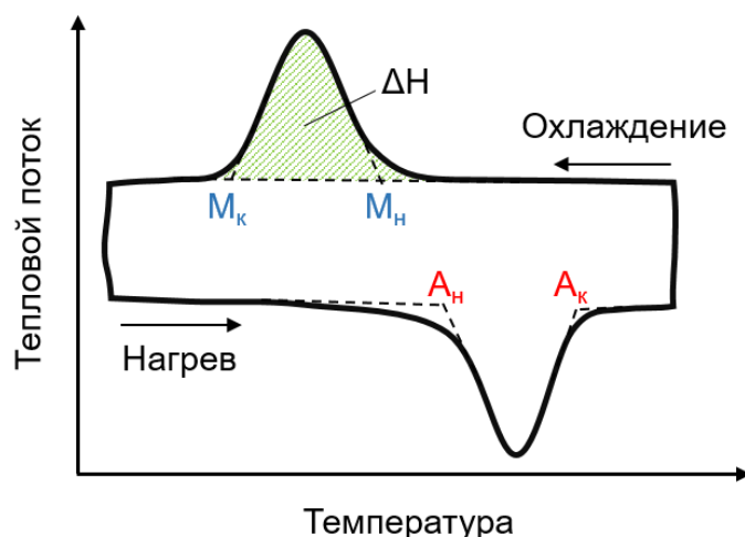
Рисунок 1.1 – Тепловые эффекты, регистрируемые при термоупругом мартенситном превращении на дифференциальном сканирующем калориметре
