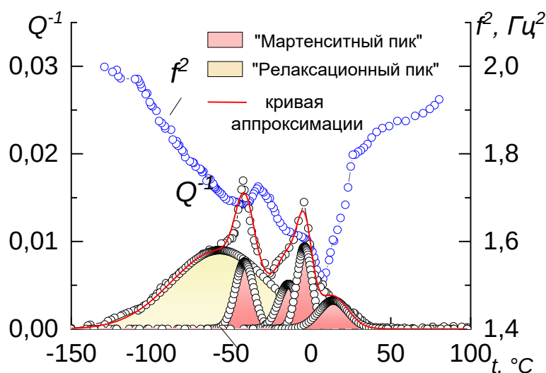
Рисунок 5.7 – ТЗВТ образца (охлаждение) после спекания (партия 1)
