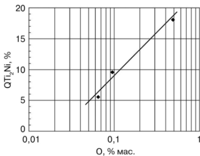
Рисунок 1.7 – Зависимость объемной доли Ti_2Ni от содержания кислорода в сплаве Ti-55,7\pm0,1Ni \% \text{ мас.} [56]
