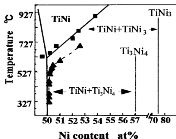
Рисунок 1.5 – Область существования метастабильных фазы Ti_3Ni_4 и TiNi_3 [10]
